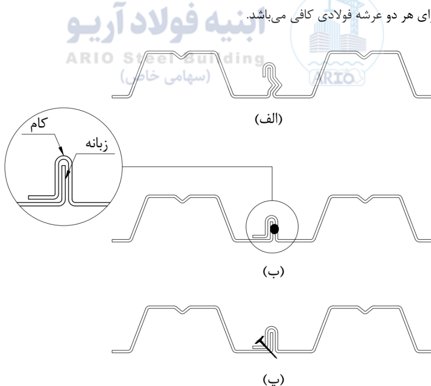
شکل ۴- انواع اتصال هم‌پوشانی جانبی عرشه‌ها بصورت کام و زبانه: الف- بست دکمه‌ای، ب- جوشی و پ- پیچی
